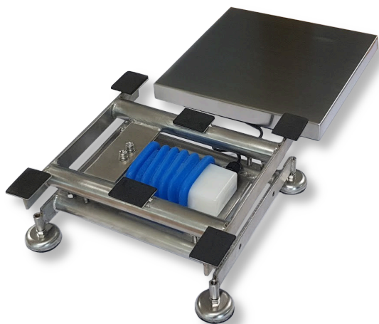
Bänkvåg BSS250x250-15 Aluminum lastcell med plastkåpa
