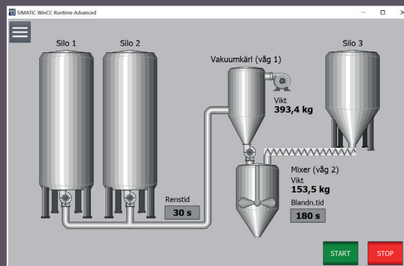
Exempel på processbild för RDS-WS
